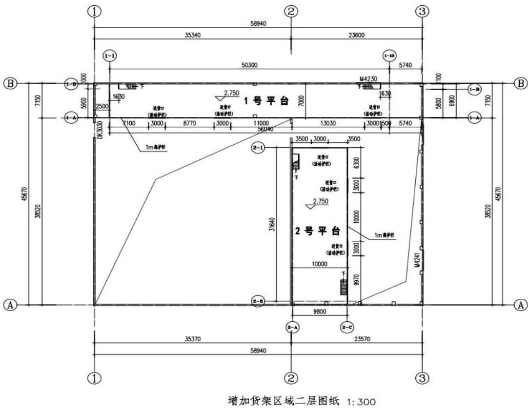
图二 招标人仓库改造规划设计图
